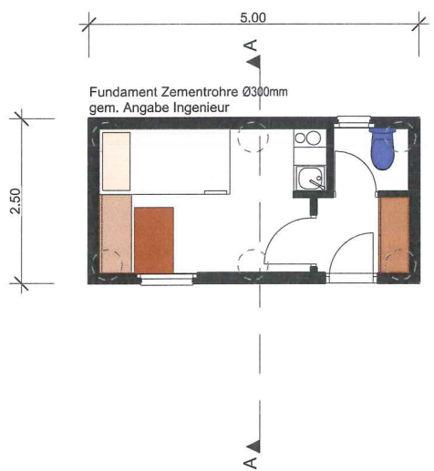
EG 1:100
