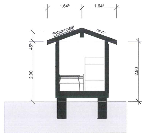
Schnitt 1:100
